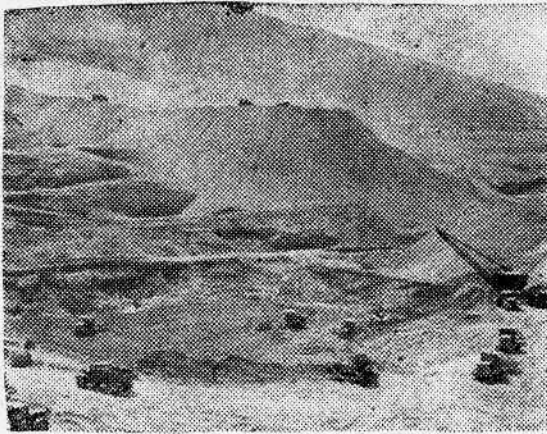
Таджикская ССР. Закончена выемка грунта из котлована под плотину. Катта-Сайского водохранилища. Эта высокогорная земляная плотина поз-
